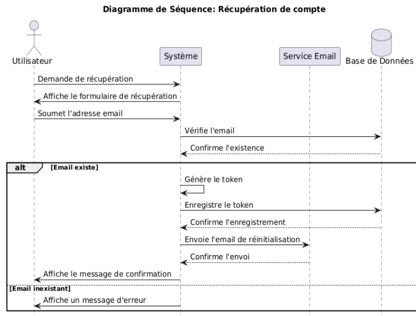
FIGURE 4.6 – Diagramme de séquence pour le scénario de récupération de compte
