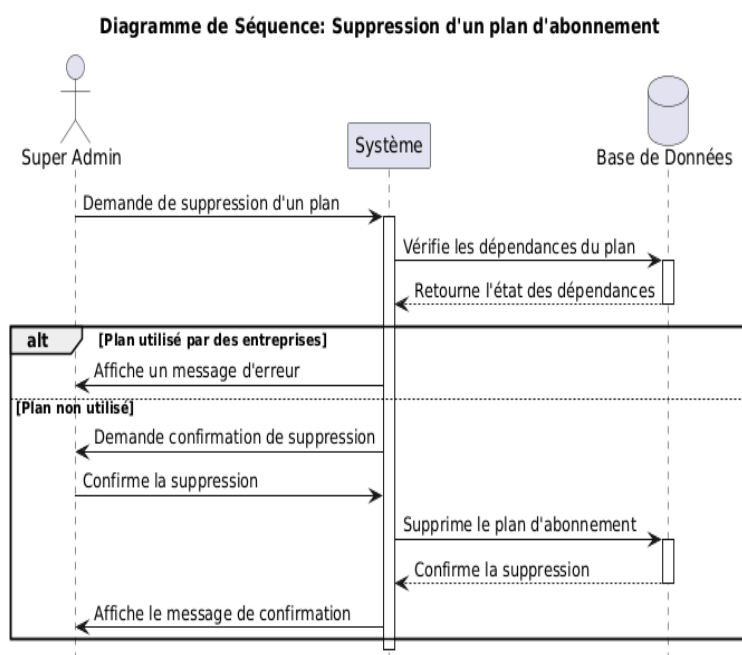
FIGURE 5.9 – Diagramme de séquence pour le scénario de suppression d'un plan d'abonnement
