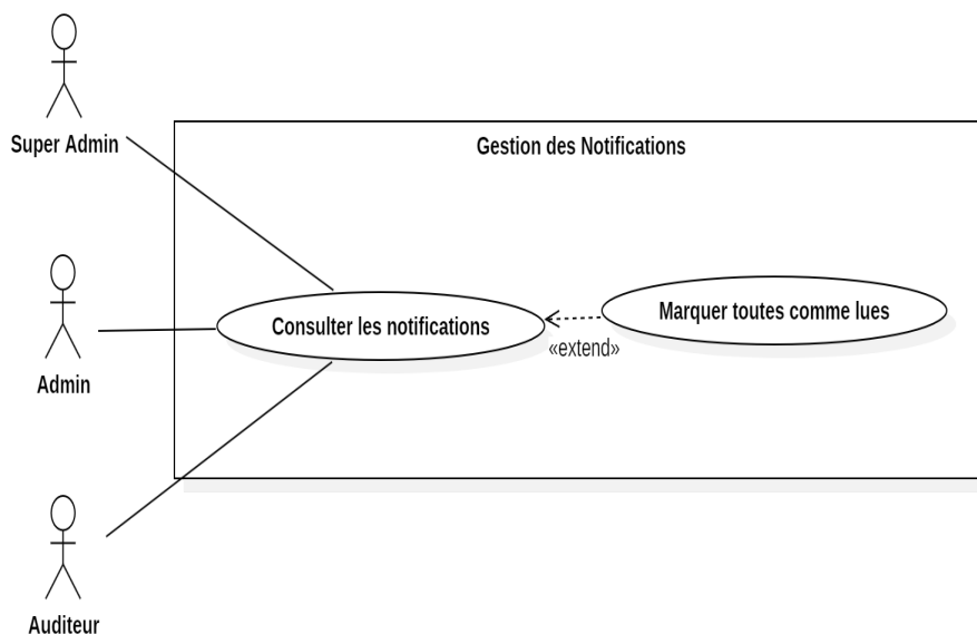
FIGURE 5.35 – Diagramme de cas d'utilisation - Gestion des notifications
