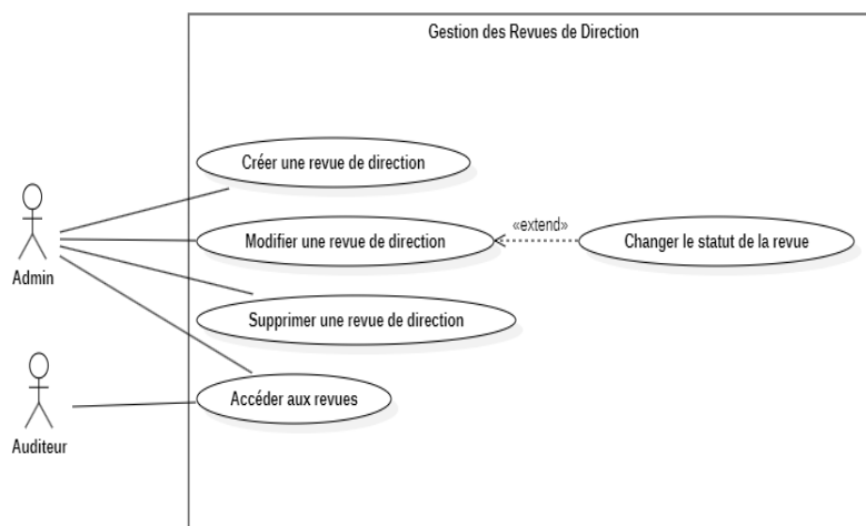
FIGURE 5.33 – Diagramme de cas d'utilisation - Gestion des revues de direction
