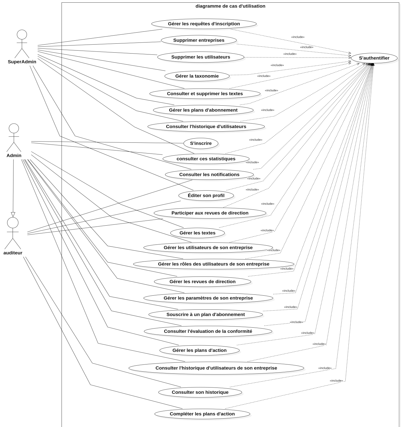
FIGURE 2.1 – Diagramme de cas d'utilisation global
