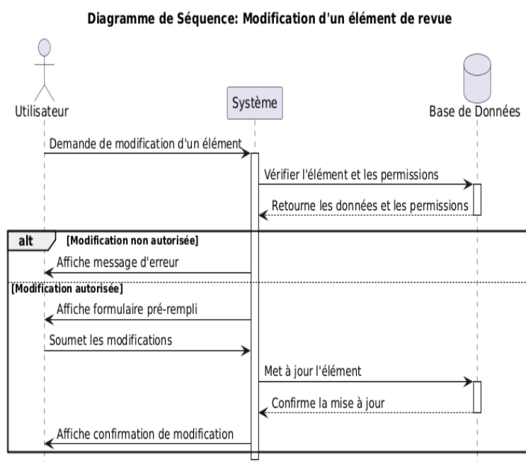
FIGURE 5.45 – Diagramme de séquence pour le scénario de modification d'un élément de revue
