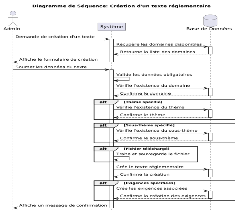
FIGURE 5.12 – Diagramme de séquence pour le scénario de création d'un texte réglementaire
