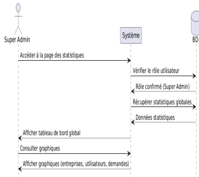
FIGURE 5.51 – Diagramme de séquence pour le scénario de consultation des statistiques globales
