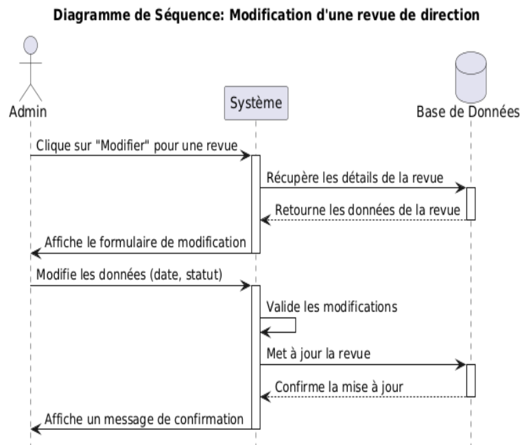
FIGURE 5.40 – Diagramme de séquence pour le scénario de modification d'une revue de direction
