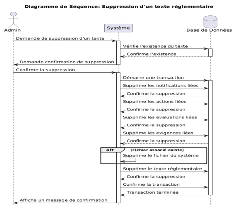
FIGURE 5.15 – Diagramme de séquence pour le scénario de suppression d'un texte réglementaire
