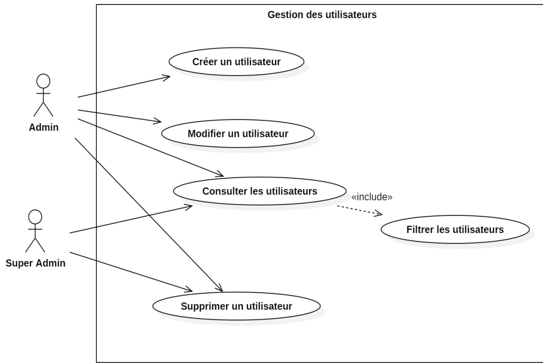
FIGURE 4.13 – Diagramme de cas d'utilisation - Gestion des utilisateurs
