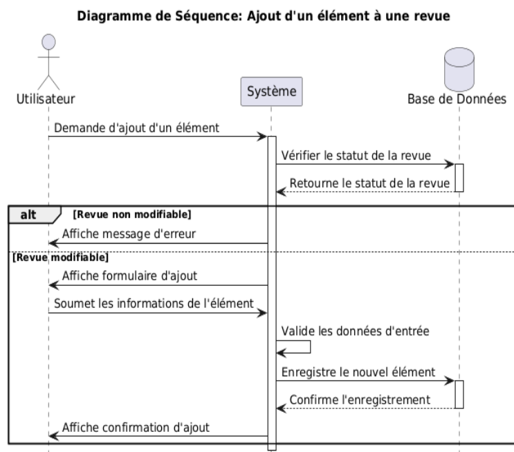
FIGURE 5.44 – Diagramme de séquence pour le scénario d'ajout d'un élément à une revue
