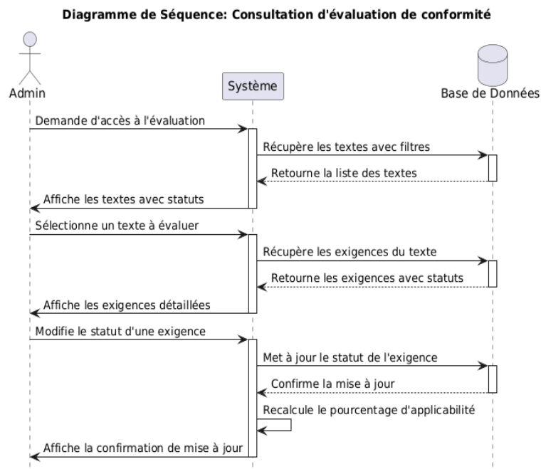
FIGURE 5.16 – Diagramme de séquence pour le scénario d'évaluation de conformité
