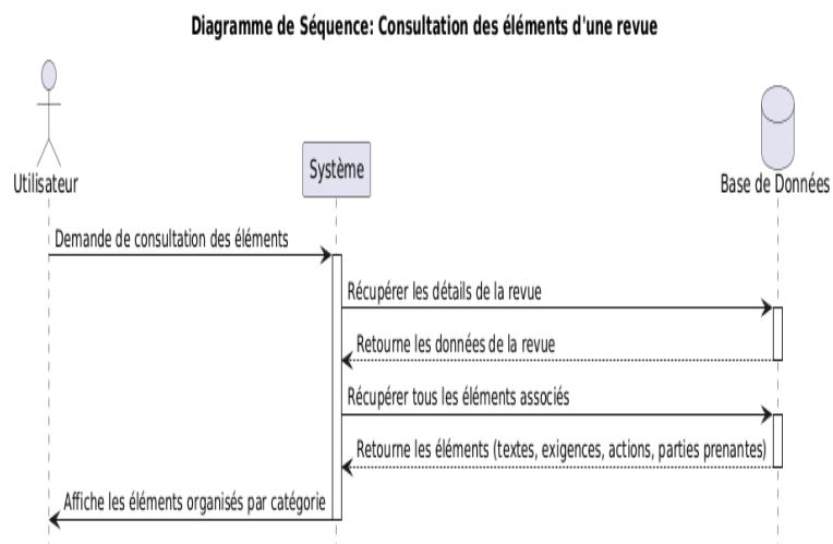
FIGURE 5.43 – Diagramme de séquence pour le scénario de consultation des éléments d'une revue
