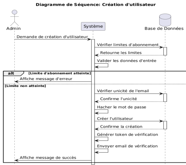
FIGURE 4.19 – Diagramme de séquence pour le scénario de création d'utilisateur
