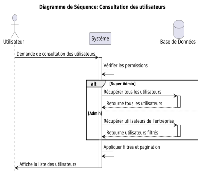
FIGURE 4.20 – Diagramme de séquence pour le scénario de consultation des utilisateurs
