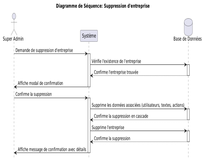
FIGURE 4.24 – Diagramme de séquence pour le scénario de suppression d'entreprise
