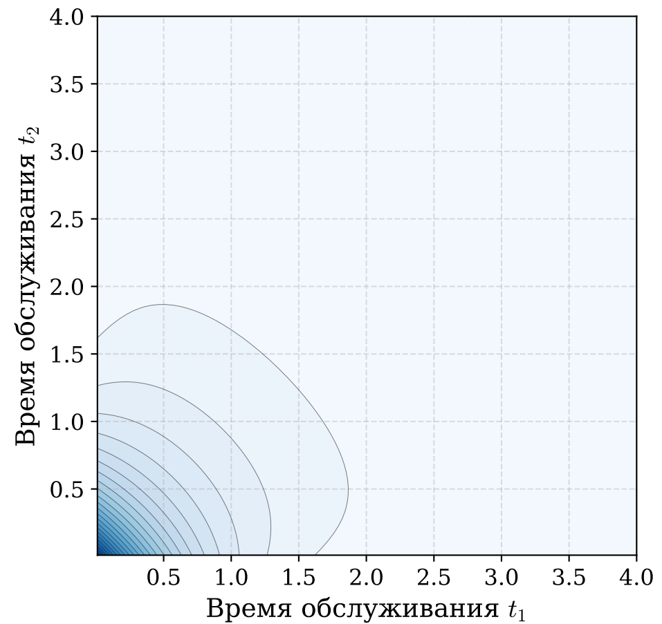
\alpha = 1 (Положительная)
