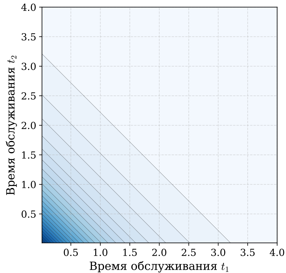
\alpha = 0 (Независимость)
