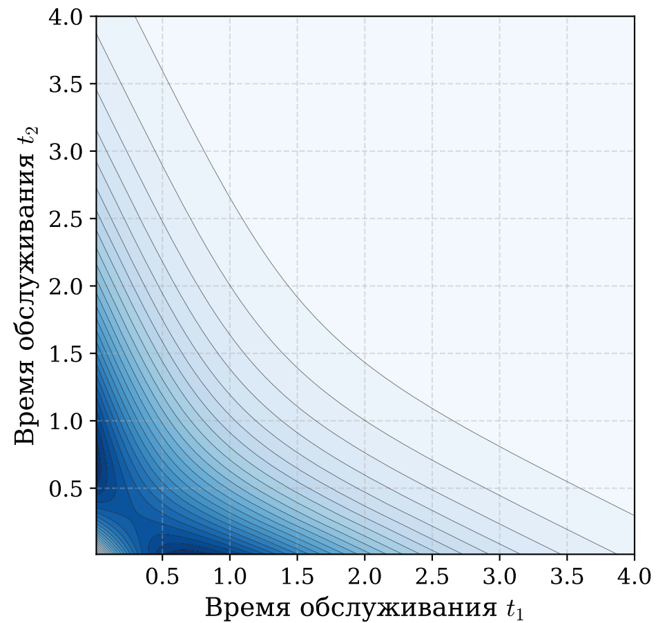
\alpha = -1 (Отрицательная)
