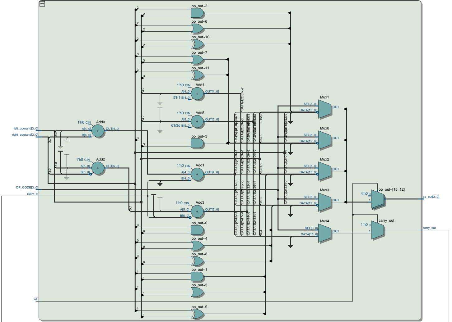
ALU:ALU_inst
