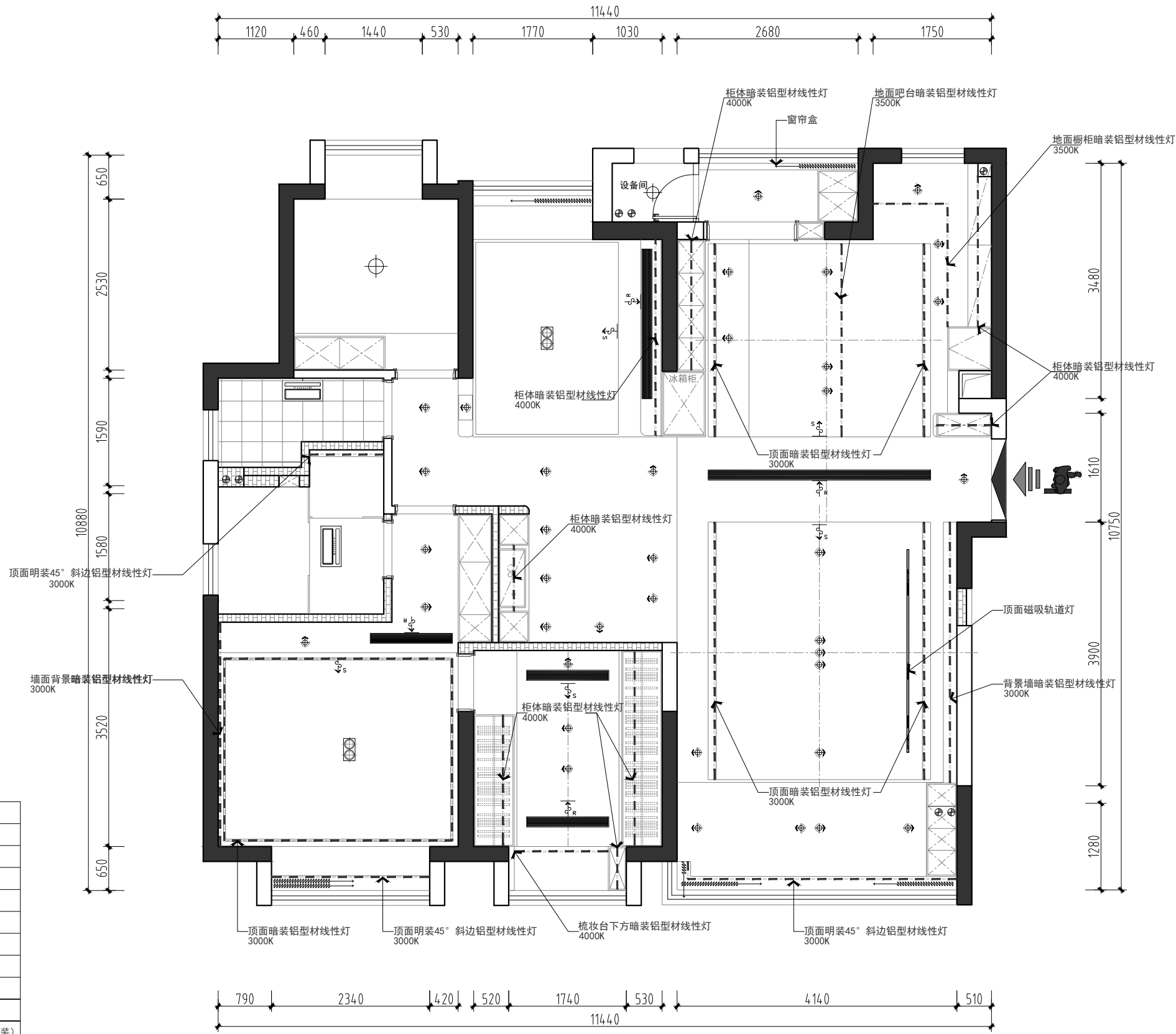
墙顶面辅助光源示意图 SCALE 1:60@A2
