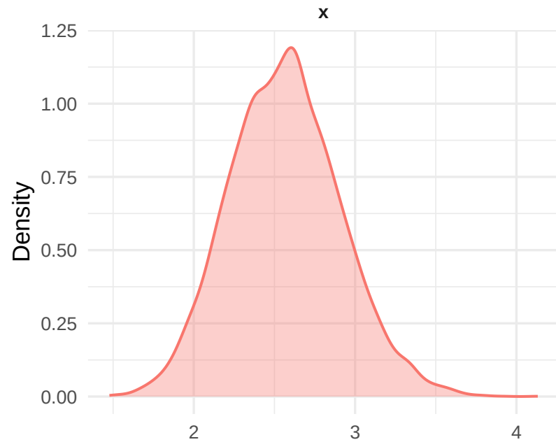
Posterior density of alpha
