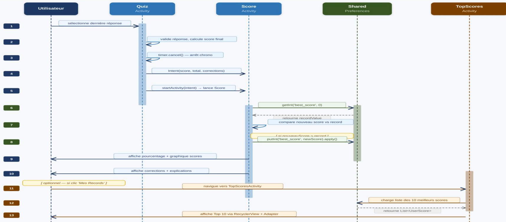
Diagramme de Séquence — Fin de Quiz — QuizApp_fj
