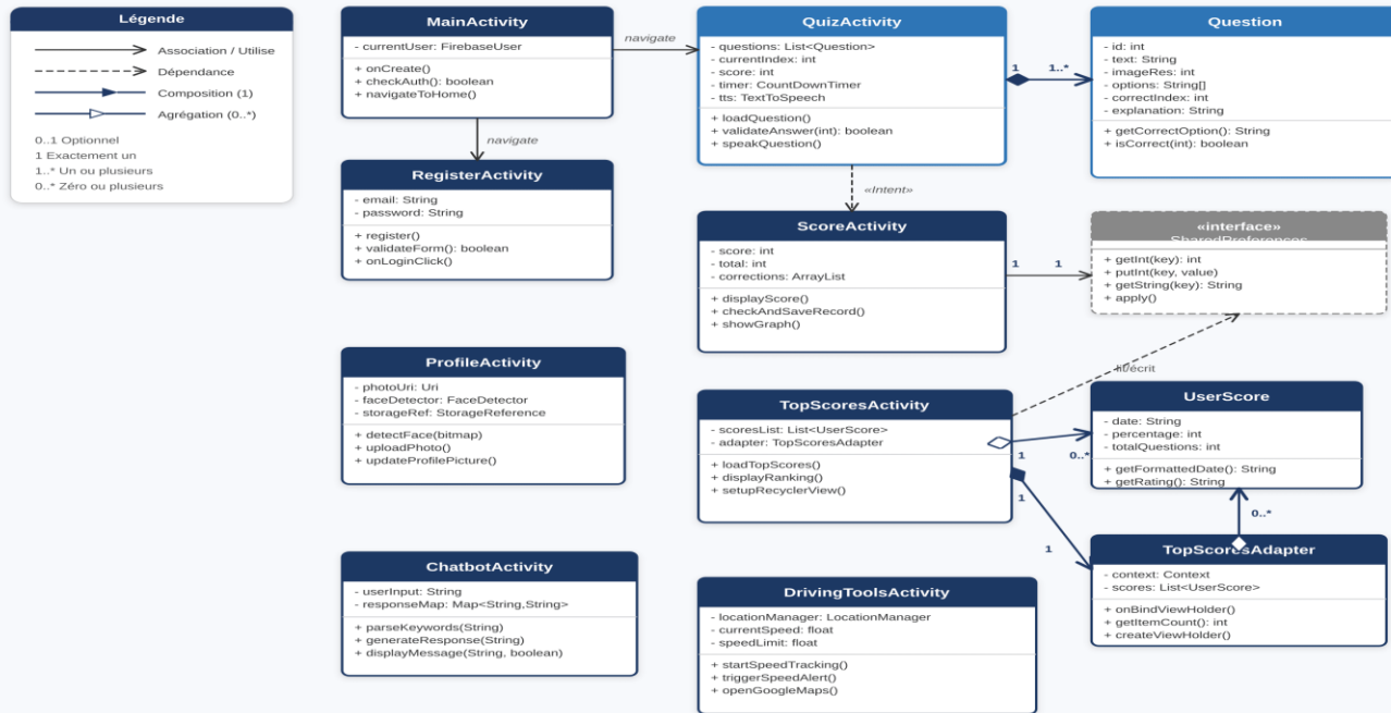
Diagramme de Classes — QuizApp_fj
