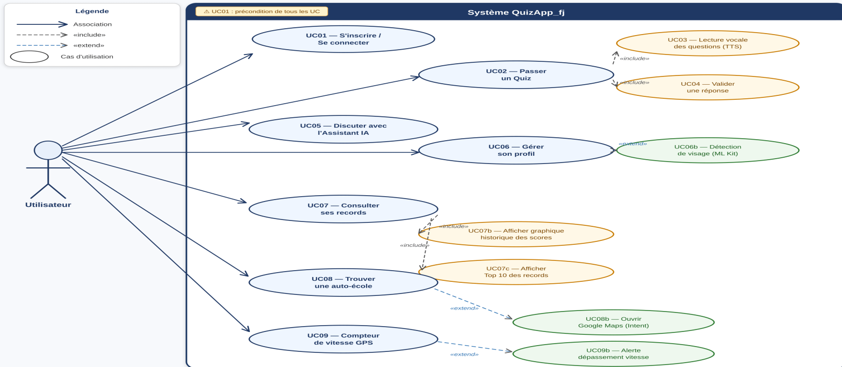
Diagramme de Cas d'Utilisation — QuizApp_fj
