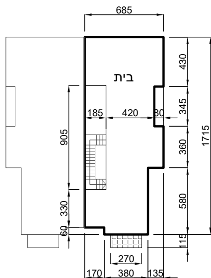
קומה א
