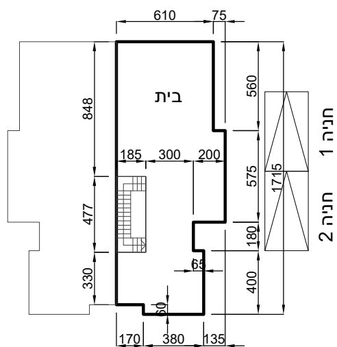
קומת קרקע
