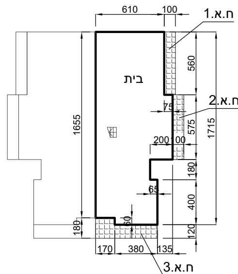
קומת מרתף
