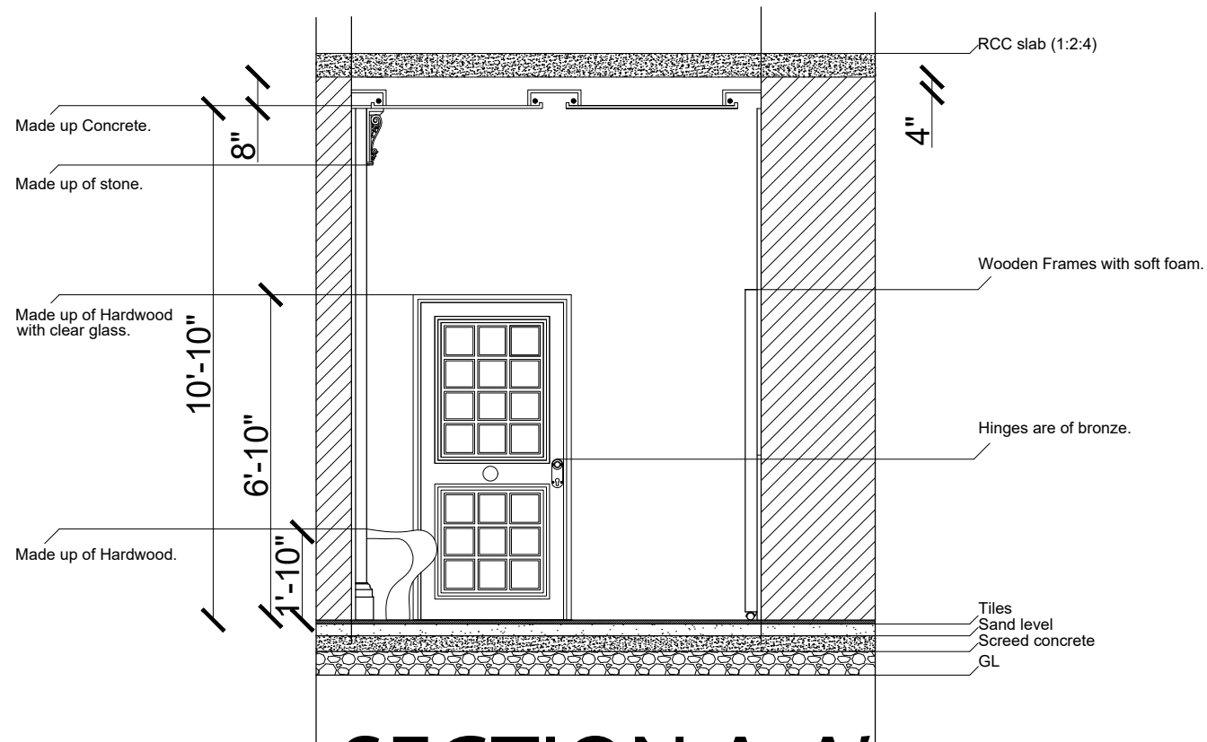
SECTION A-A'
