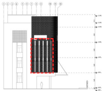
Right Elevation
