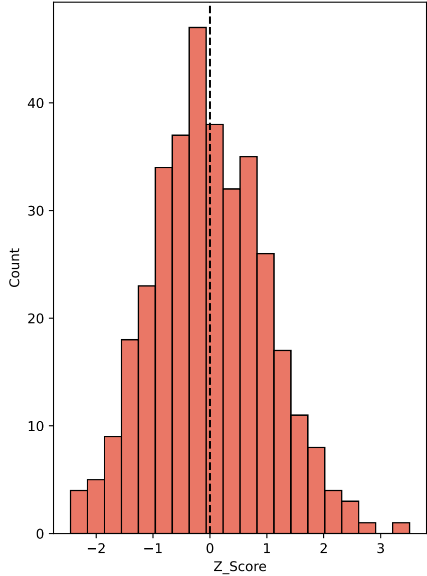
Z-score Escuelas: Lengua
