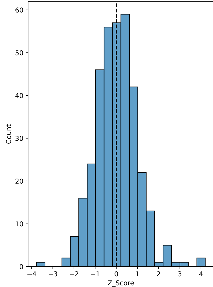
Z-score Escuelas: Matemática
