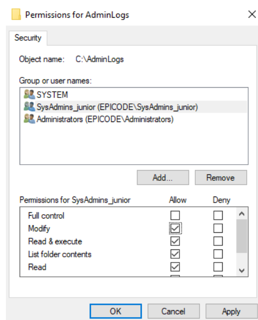
Fig. 3 — Permessi NTFS su C:\AdminLogs (gruppo SysAdmins_Junior)
