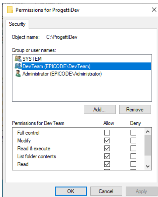
Fig. 2 — Permessi NTFS su C:\ProgettiDev (gruppo DevTeam)
