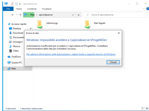
Fig. 8 — Frank tenta di aprire ProgettiDev: il suo gruppo non ha permessi di accesso
