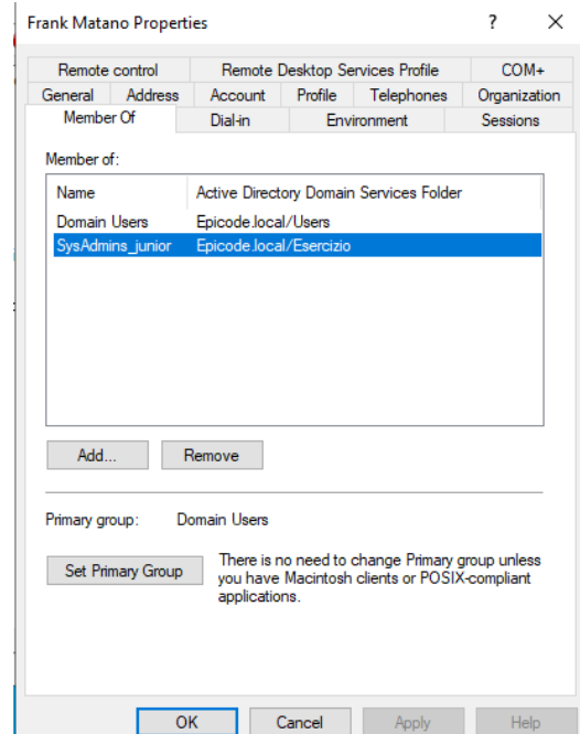
Fig. 7 — Frank Matano, membro del gruppo SysAdmins_Junior
