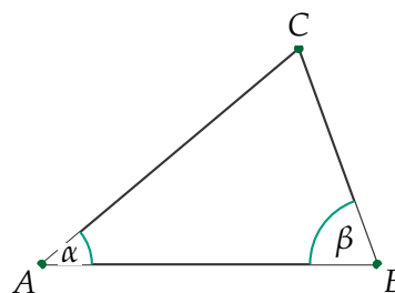
Caso 2: BC < AC
