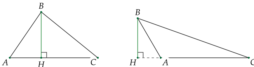
Izquierda: \angle A agudo y H en el rayo \overrightarrow{AC} . Derecha: \angle A obtuso y H en el rayo opuesto, con H - A - C .
