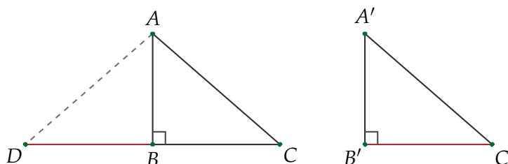
Criterio hipotenusa-cateto: se copia el cateto \overline{B'C'} al otro lado de B , obteniendo el isósceles \triangle ADC .
