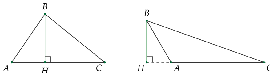
Izquierda: \angle A agudo y H en el rayo \overrightarrow{AC} . Derecha: \angle A obtuso y H en el rayo opuesto, con H - A - C .
