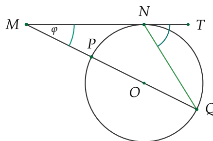
Parte II: la cuerda \overline{NQ} produce el triángulo \triangle MNQ , cuyo ángulo exterior en N es semi-inscrito.
