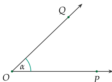
El ángulo \angle POQ , de vértice O y lados \overrightarrow{OP} y \overrightarrow{OQ} .
