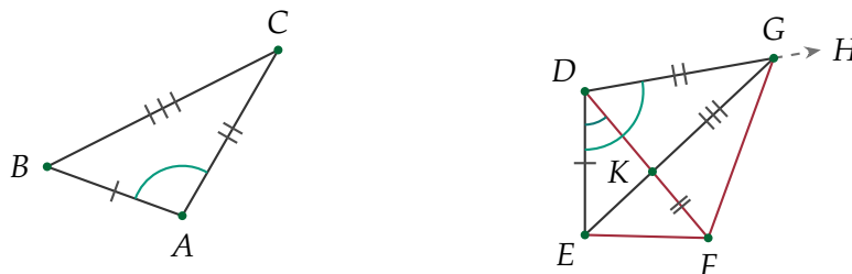
El triángulo \triangle DEG es una copia de \triangle ABC ; los segmentos \overline{DF} y \overline{EG} se cortan en K .
