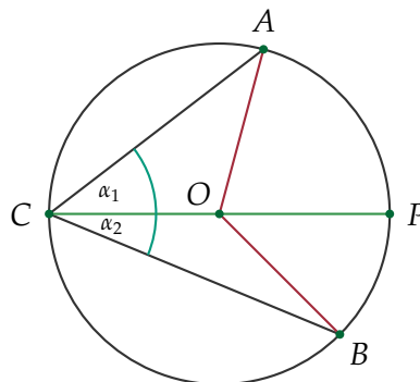
Caso 2: el diámetro \overline{CP} parte el ángulo en dos ángulos del caso 1.
