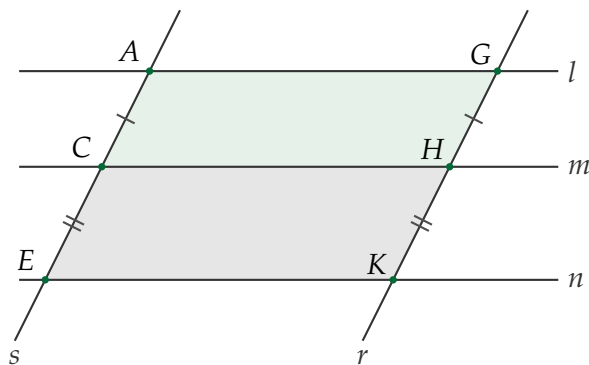
Caso 2: con las secantes paralelas los trozos correspondientes son lados opuestos de paralelogramos, luego congruentes, y la proporción es trivial.
