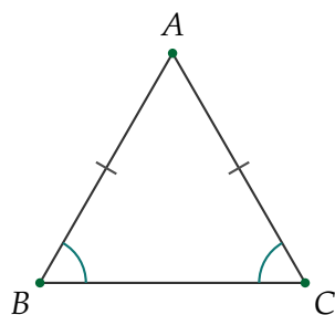
isósceles desde A: \hat{B} \cong \hat{C}
