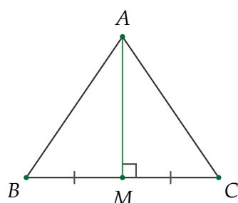
caso 1: mediana = altura
