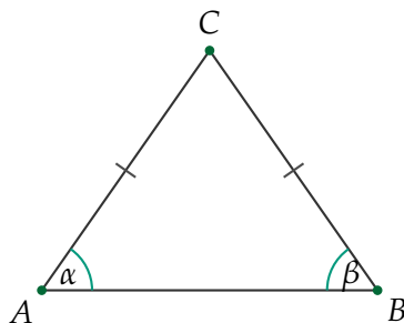
Caso 1: BC = AC
