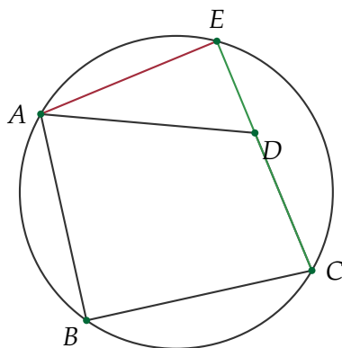
Caso A: D interior. El lado \overline{CD} se prolonga hasta cortar a \mathcal{C} en E y se traza la cuerda auxiliar \overline{AE} .
