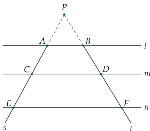
Caso 1: dos aplicaciones del teorema de Thales en el triángulo, una en \triangle PEF y otra en \triangle PCD , dan las dos proporciones que se empalman por el cociente PC/PD .
