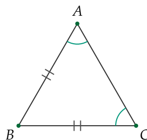
isósceles desde B: \hat{A} \cong \hat{C}
