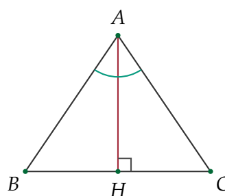
caso 2: altura = bisectriz
