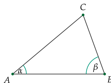
Caso 2: BC < AC
