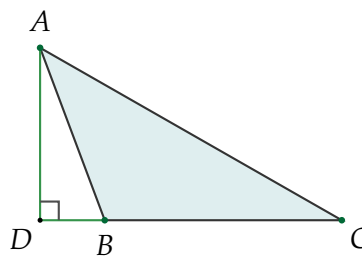
Caso 3: B entre D y C
