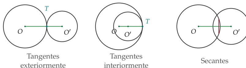
Las circunferencias con uno o dos puntos comunes: las dos tangencias y el caso secante, con su cuerda común en rojo.
