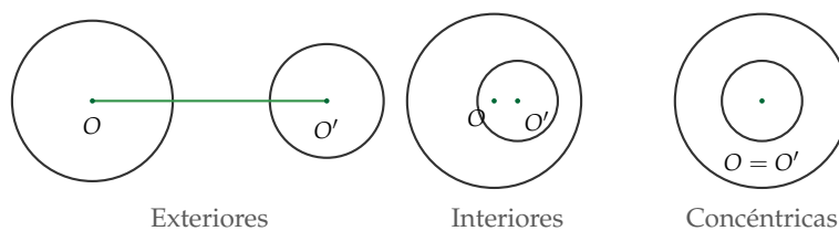
Las circunferencias sin puntos comunes: exteriores, interiores y el caso particular de las concéntricas.
