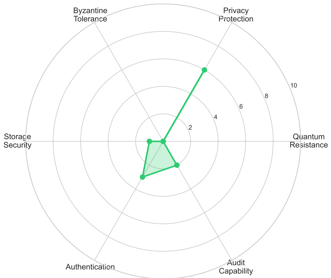
DP-FedAvg
