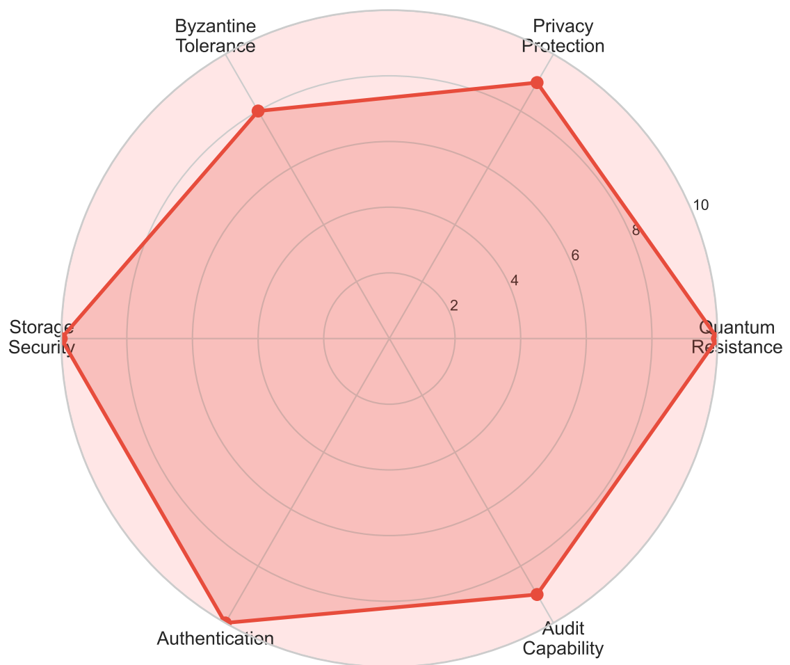
QFLARE
