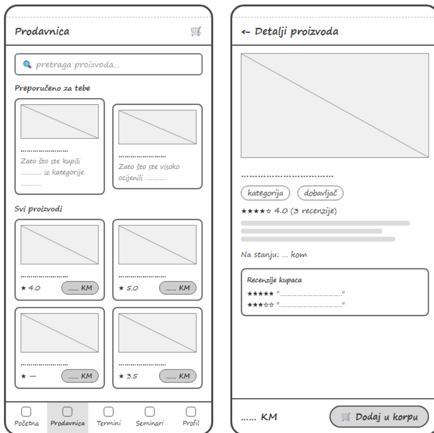
Slika 13: Prodavnica sa preporukama i detalji proizvoda
