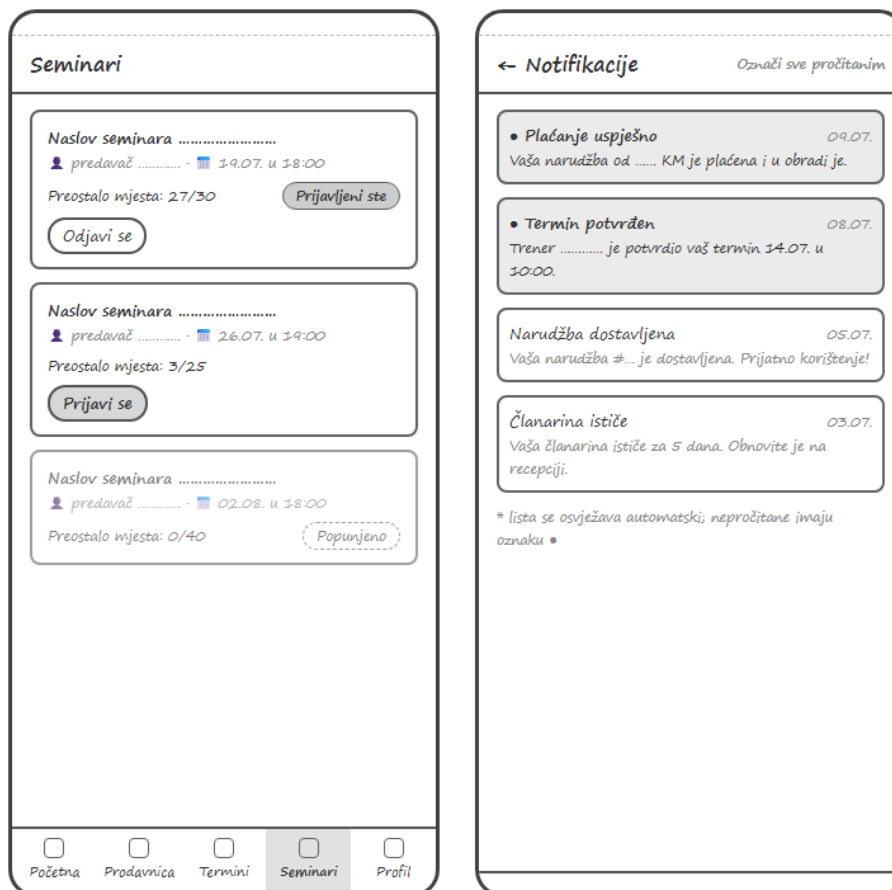
Slika 17: Seminari i notifikacije
