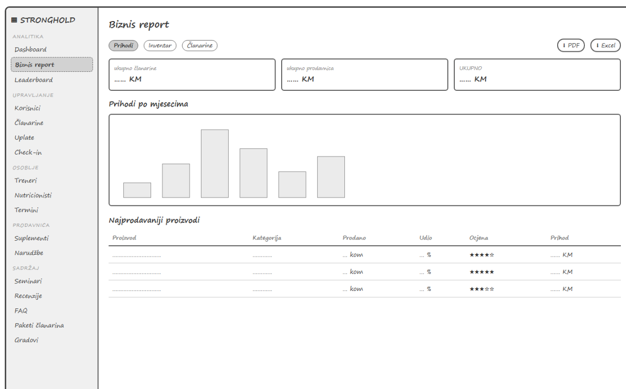
Slika 3: Biznis report, tab Prihodi
