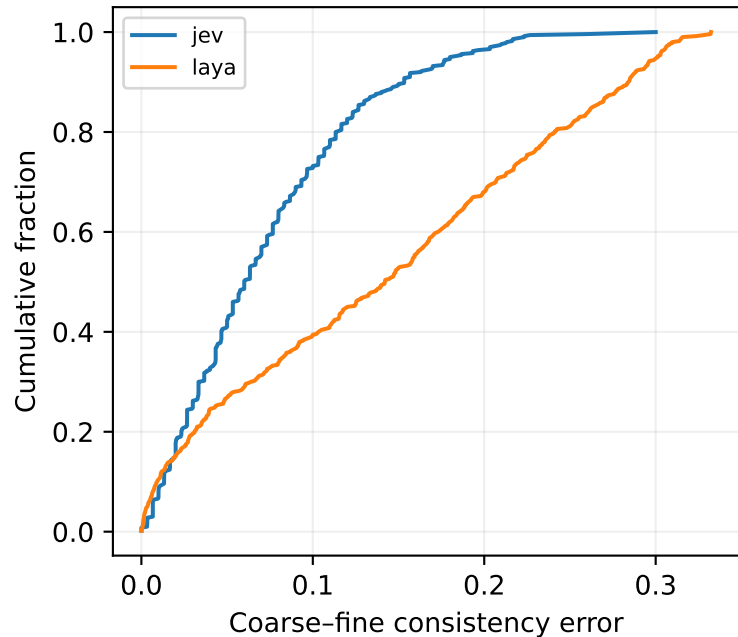
TREC
