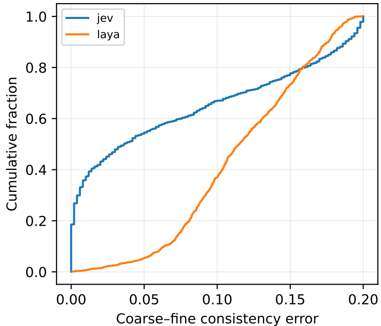
CLINC
