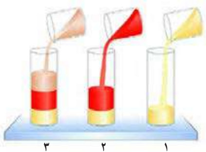
شکل ۱۳- نحوه تشکیل توالی از لایه‌های رسوبی
