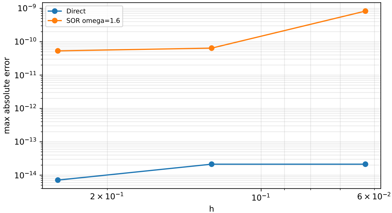
A: max error vs mesh size
