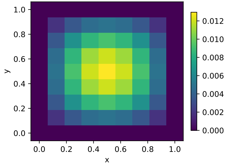
Absolute Error
