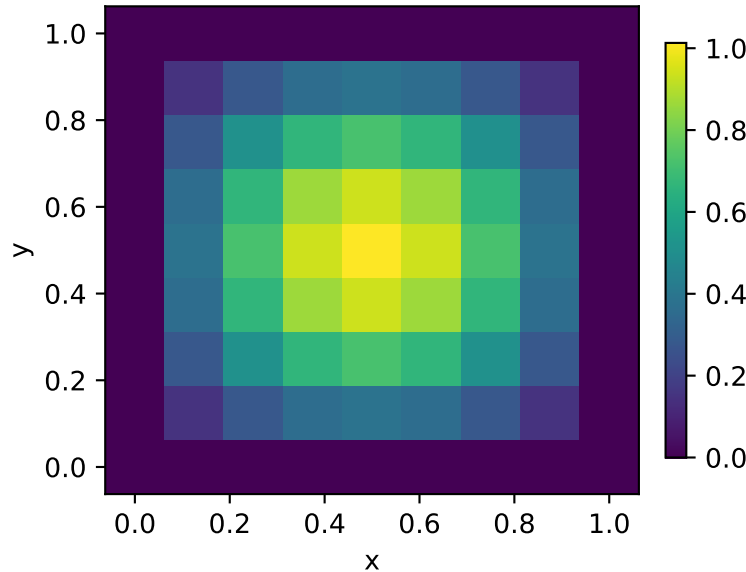
Numerical
