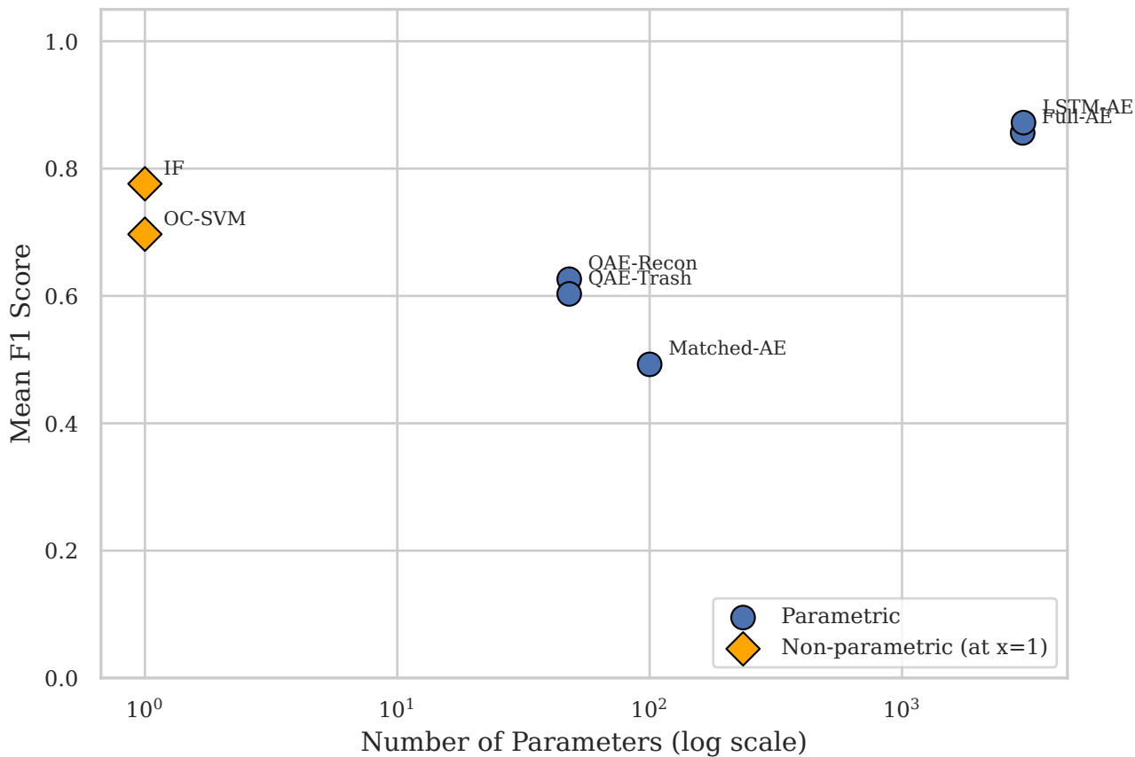
Parameter Count vs. Mean F1 Score
