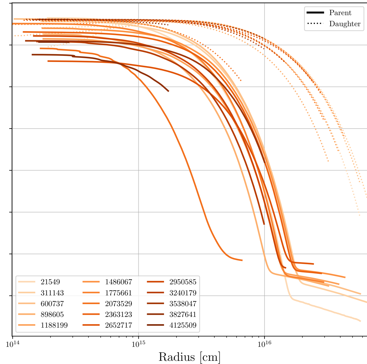
HCN - CN
