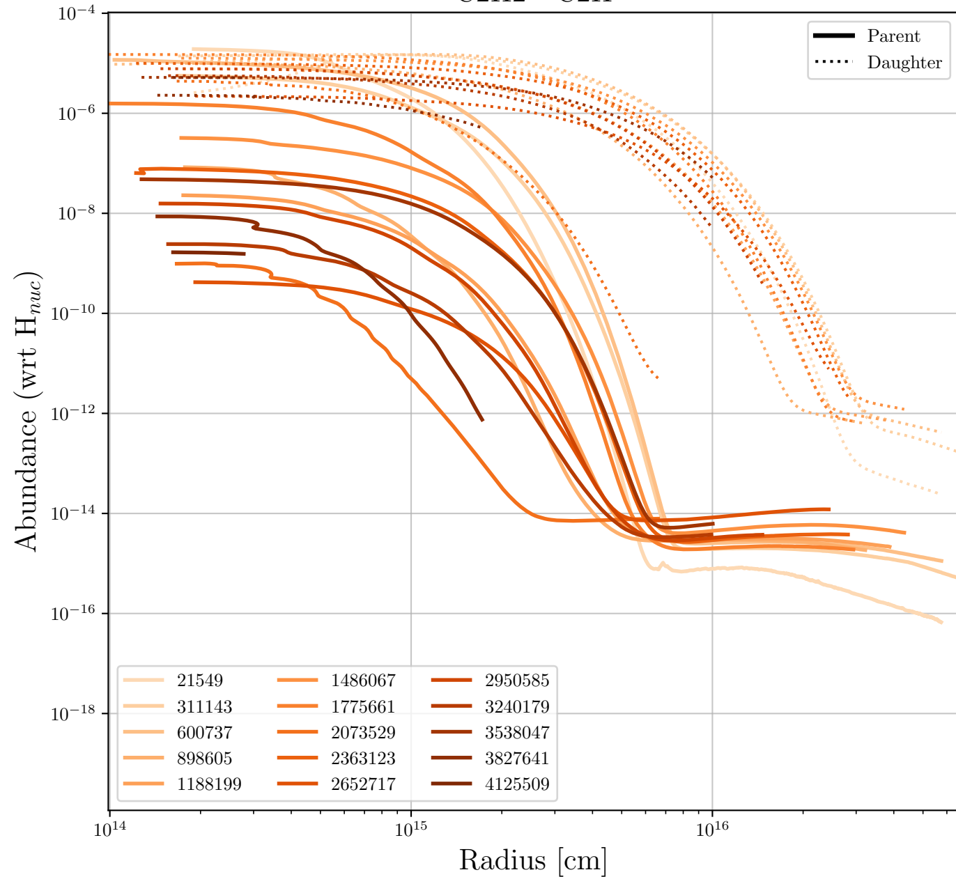
C2H2 - C2H
