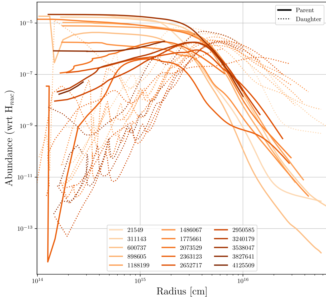
C2H2 - C2H
