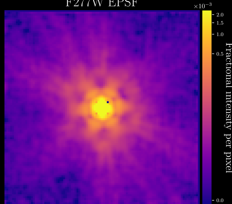
F277W EPSF
