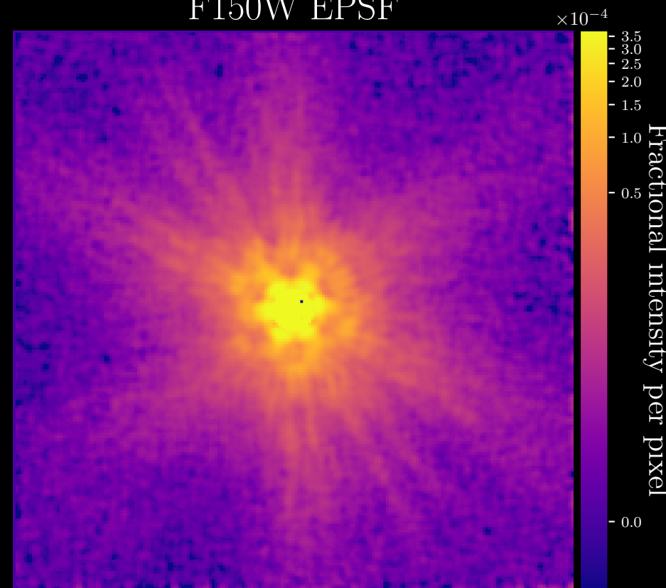
F150W EPSF
