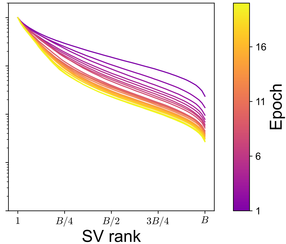
MNIST
