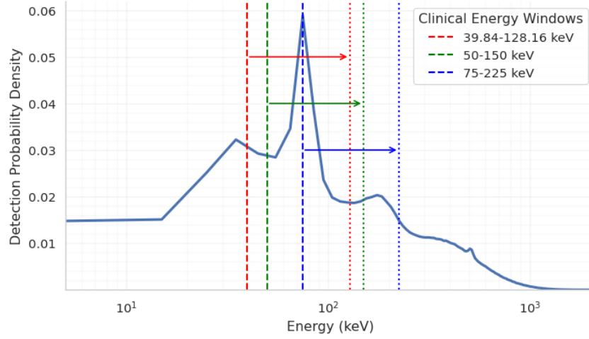
(b) Detected spectrum (10 cm, AnyScan).
