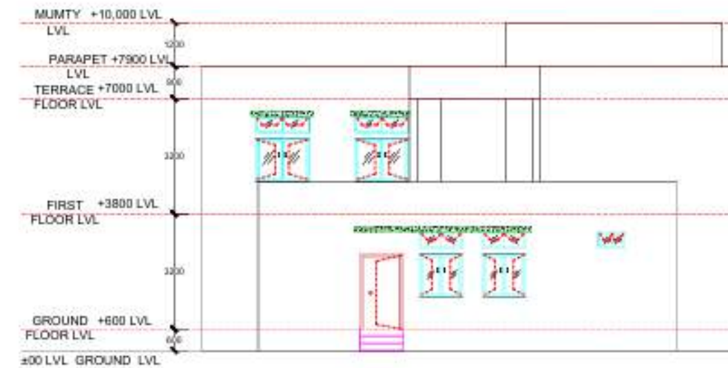
ELEVATION D-D'
