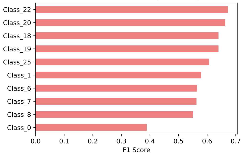
Bottom 10 Classes (F1 Score)
