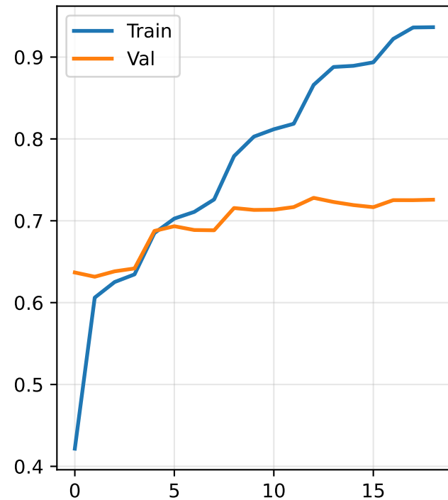
F1 Score
