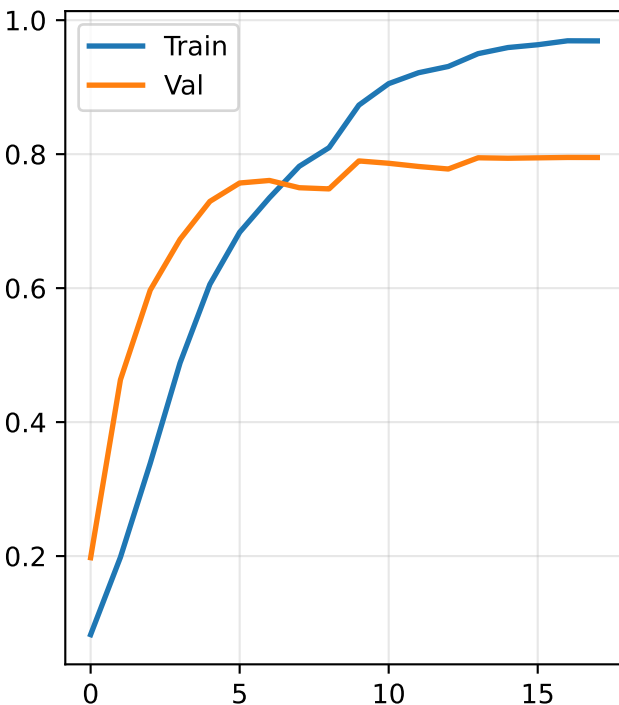
F1 Score
