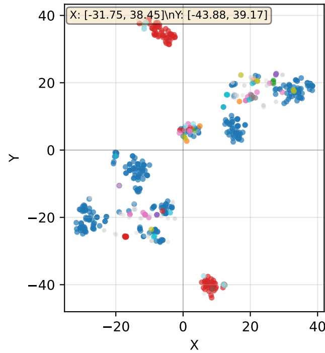
PaCMAP - Raw
