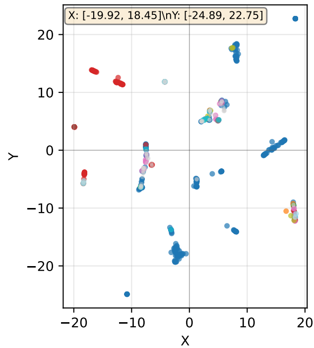
LocalMAP - Raw
