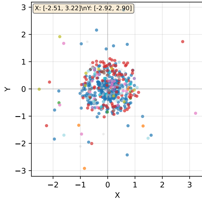
LocalMAP - Raw
