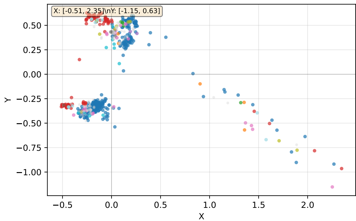
UMAP - Raw
