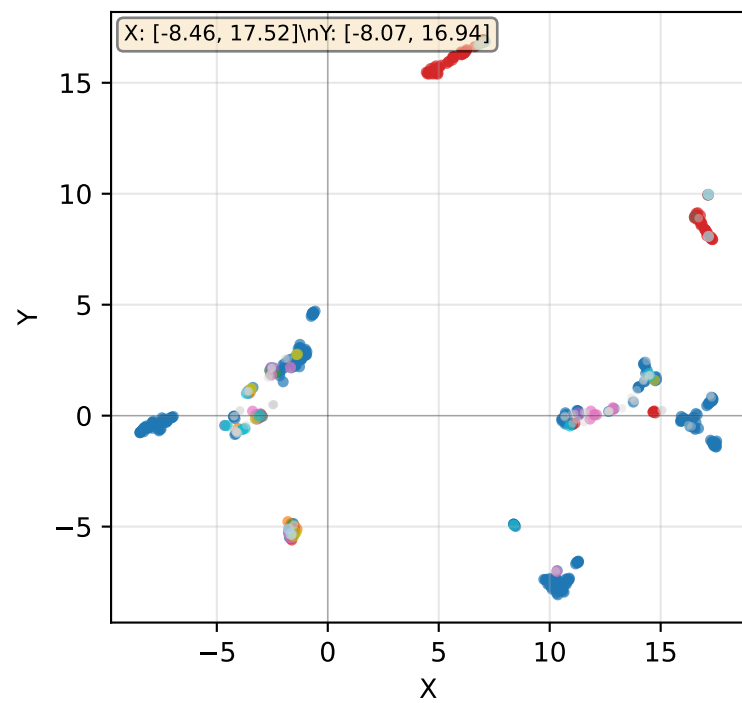
t-SNE - Raw
