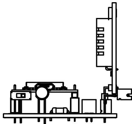
COMMAND MODULE ( 1 : 1 )
