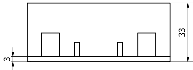
BODY ( 1 : 1 )
