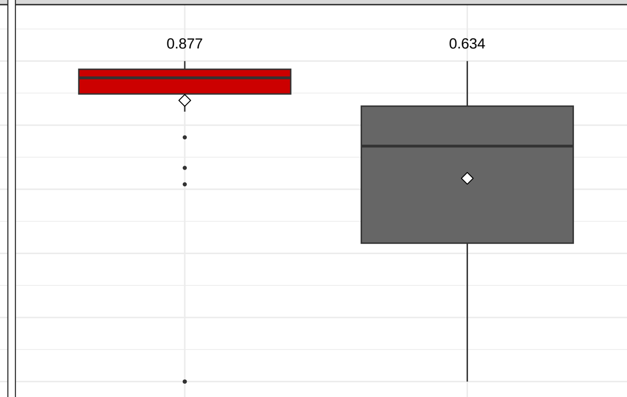
F1 Score
