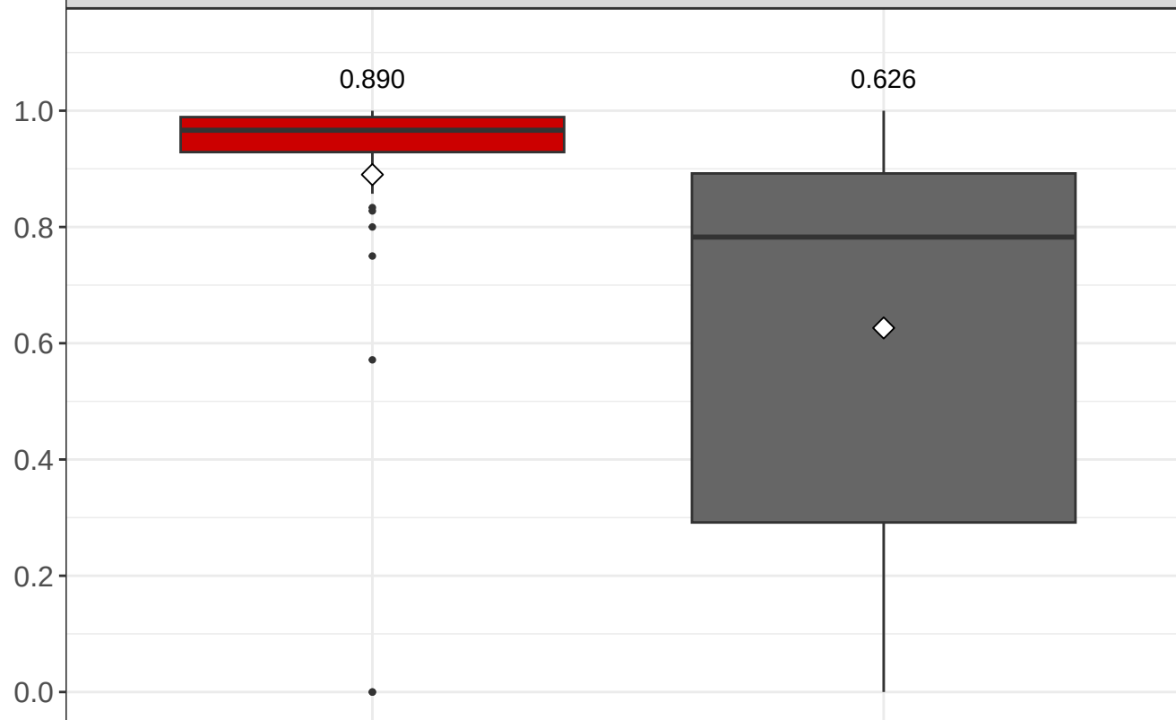
Precision
