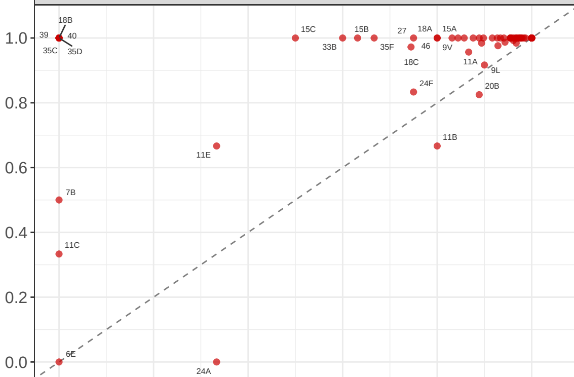
Precision
