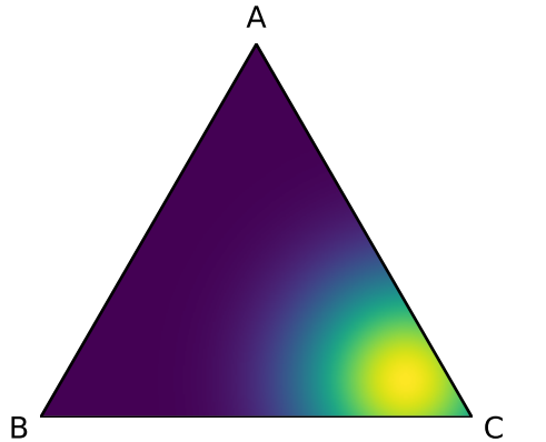
(d) Out-of-distribution
