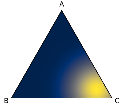
(d) Out-of-distribution
