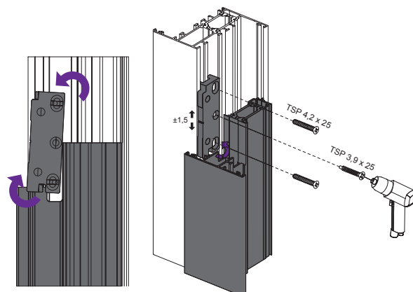
Montaggio / Assembly
