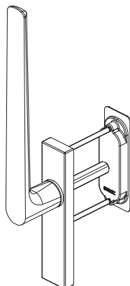
MANIGLIONE ALZANTE, CON MANIGLIA DI TRASCIMENTO QUADRO 10 MM (AS300-HS) - LIFT & SLIDE HANDLE WITH PULL HANDLE PIN 10 MM (AS300-HS)
