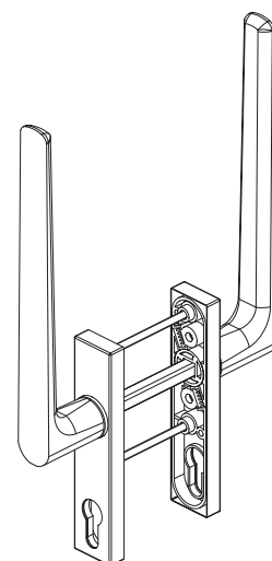
MANIGLIONE DOPPIO ALZANTE QUADRO 10 MM (AS300-HS) - LIFT & SLIDE DOUBLE HANDLE PIN 10 MM (AS300-HS)
