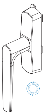
CREMONESE - CREMONE BOLT
