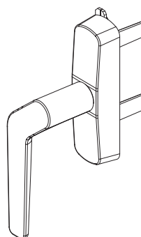
CREMONESE CON MANICO DISASSATO DESTRO - CREMONE BOLT WITH RIGHT CRANK HANDLE
