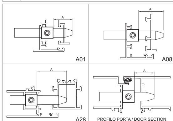
Anta Cava Erre Erre Groove Sash
