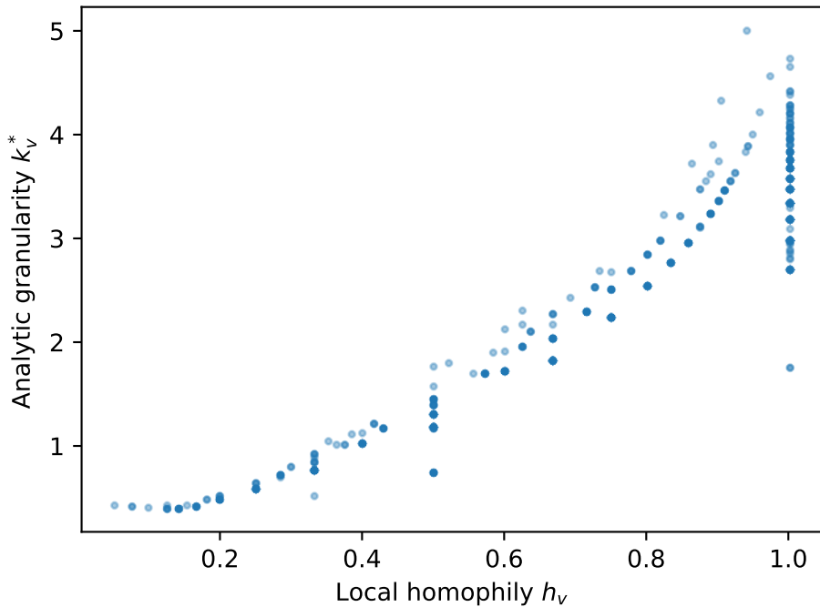
Citeseer — r=0.963
