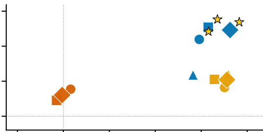
Hivemind diversity
