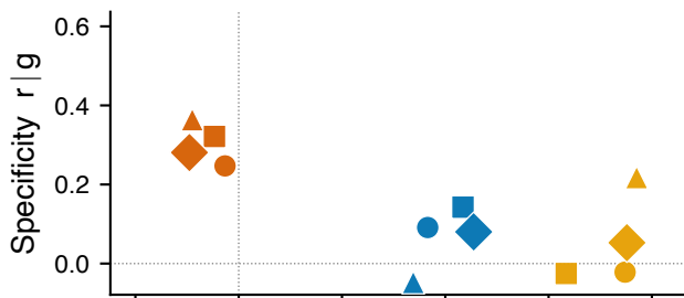
Arena CW
