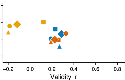
Hivemind diversity
