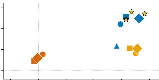
EQ-Bench CW
