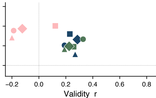
Hivemind diversity
