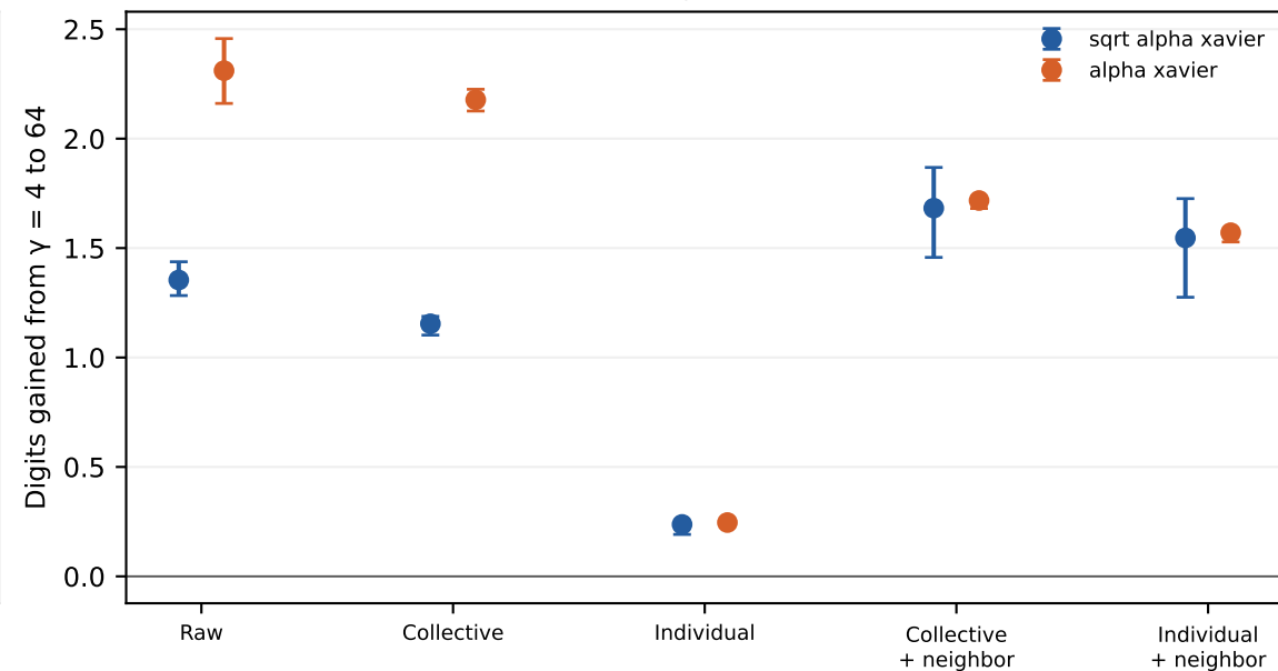
Runge · ADAM
