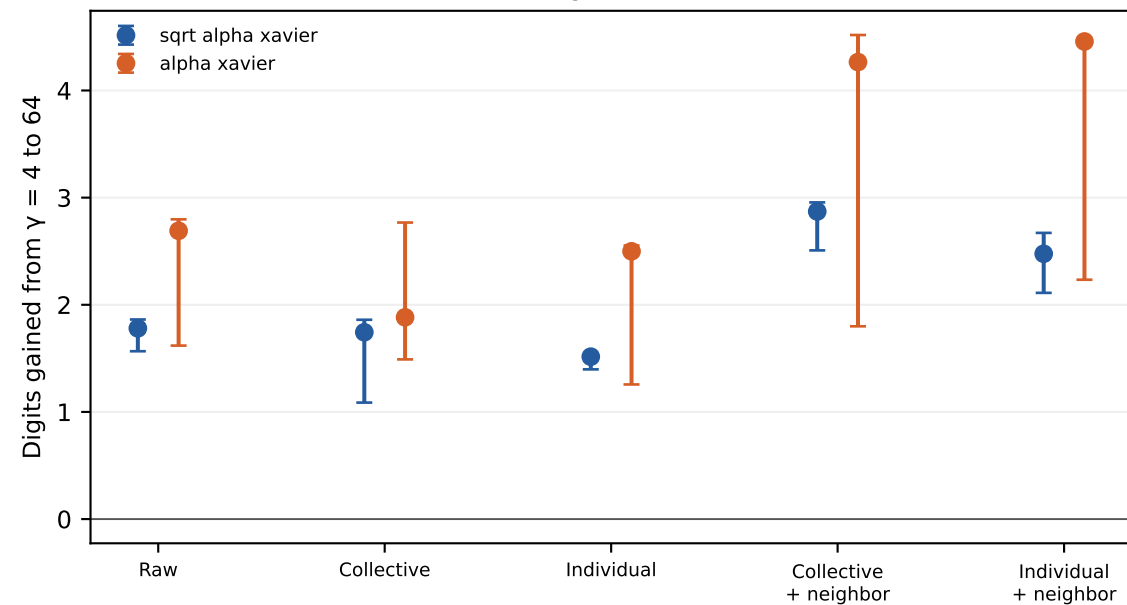
Runge · ADAM
