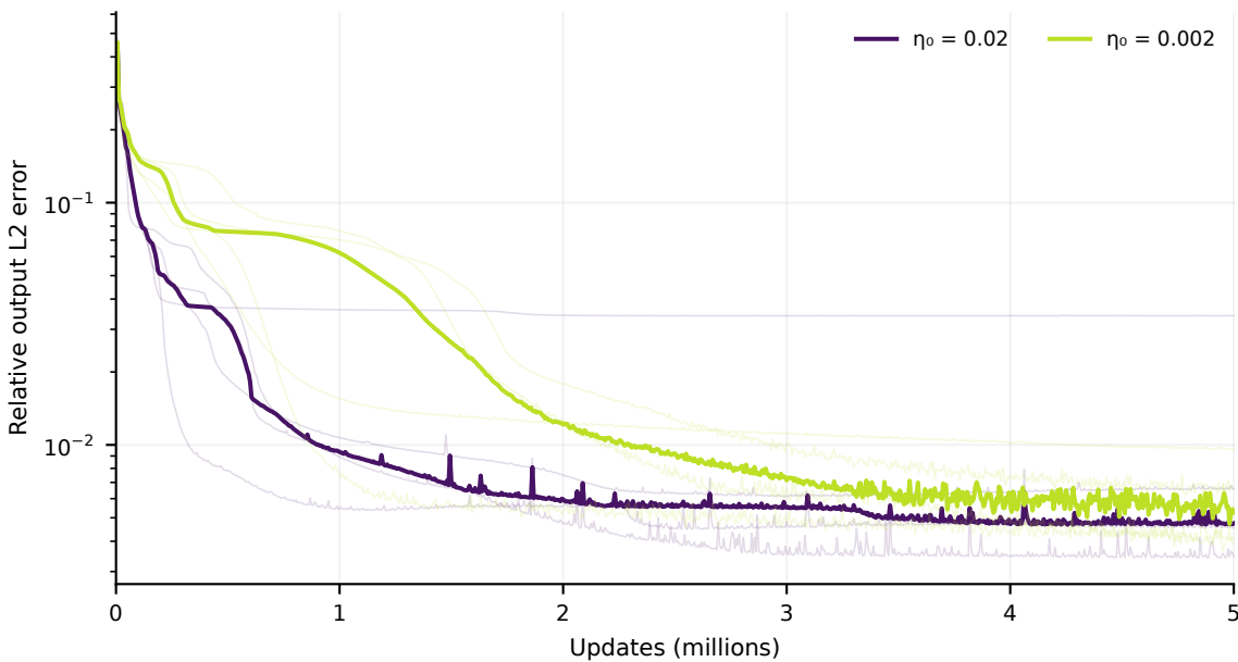
GD · constant
