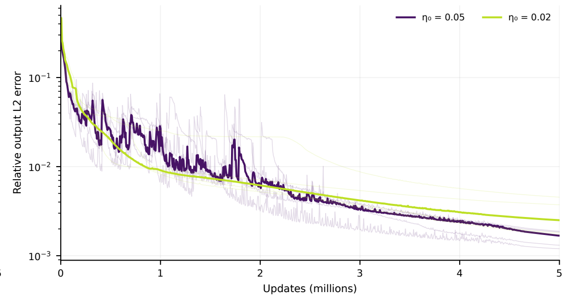
GD · cosine
