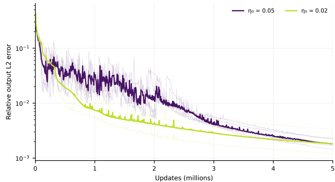
GD · cosine
