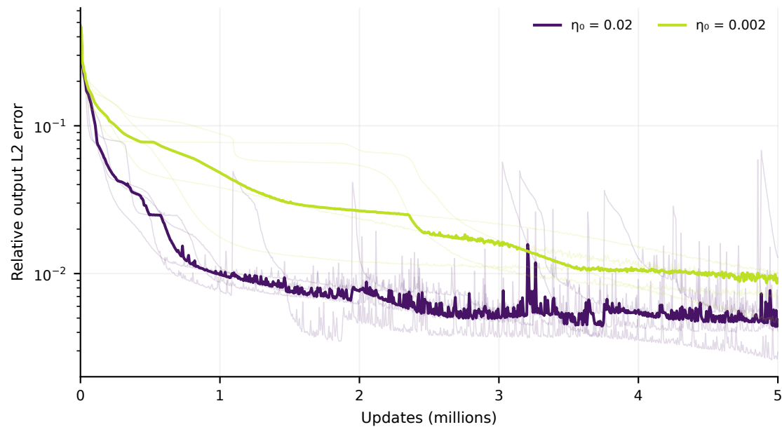
GD · constant
