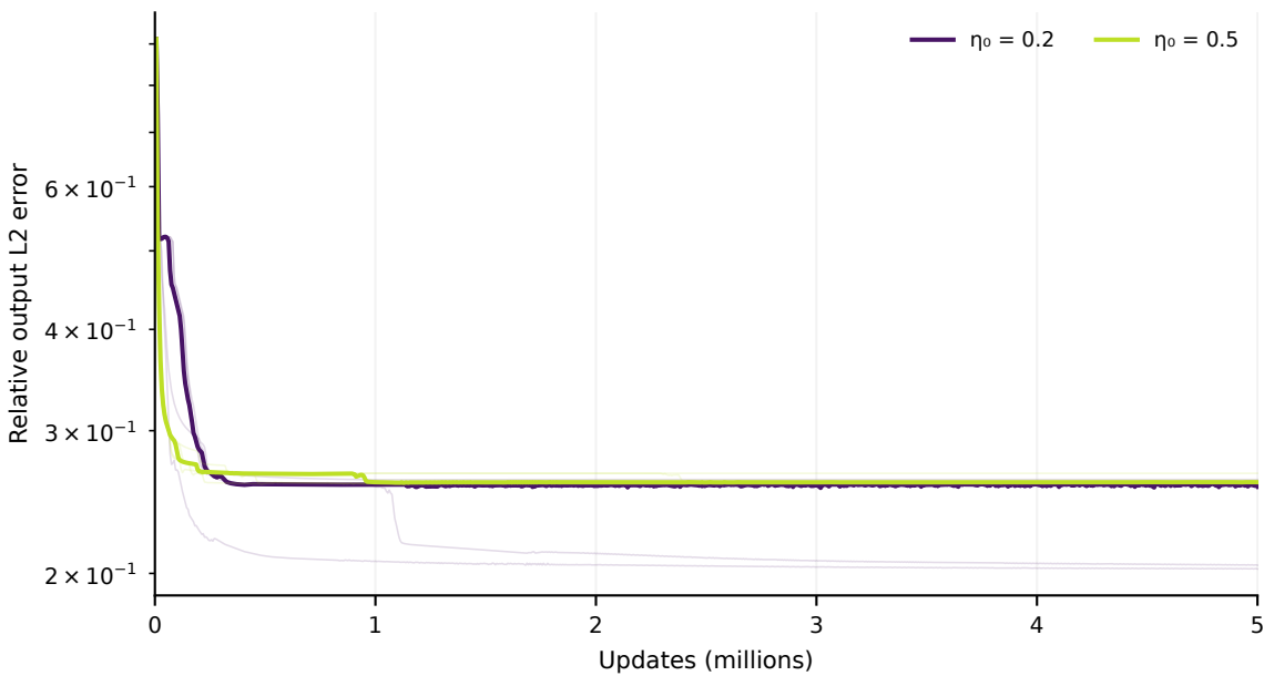
GD · constant
