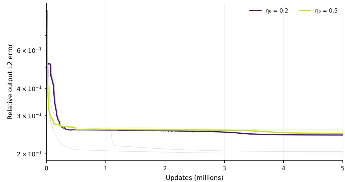
GD · cosine
