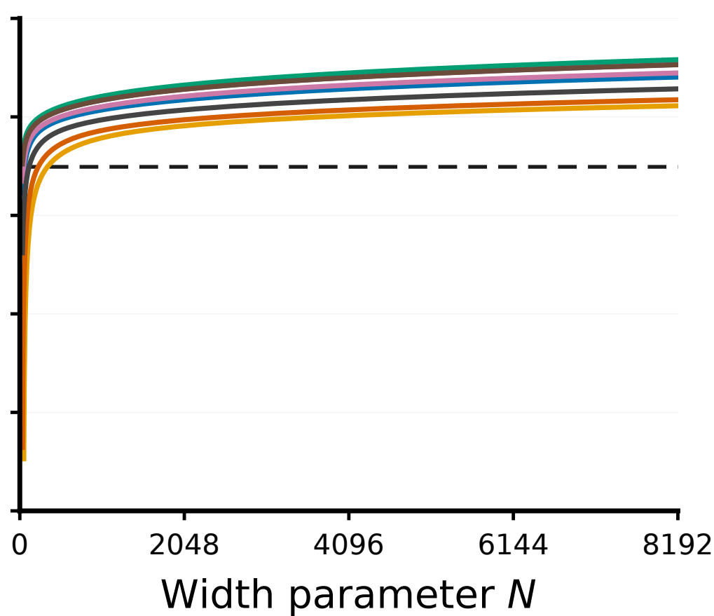
GELU
