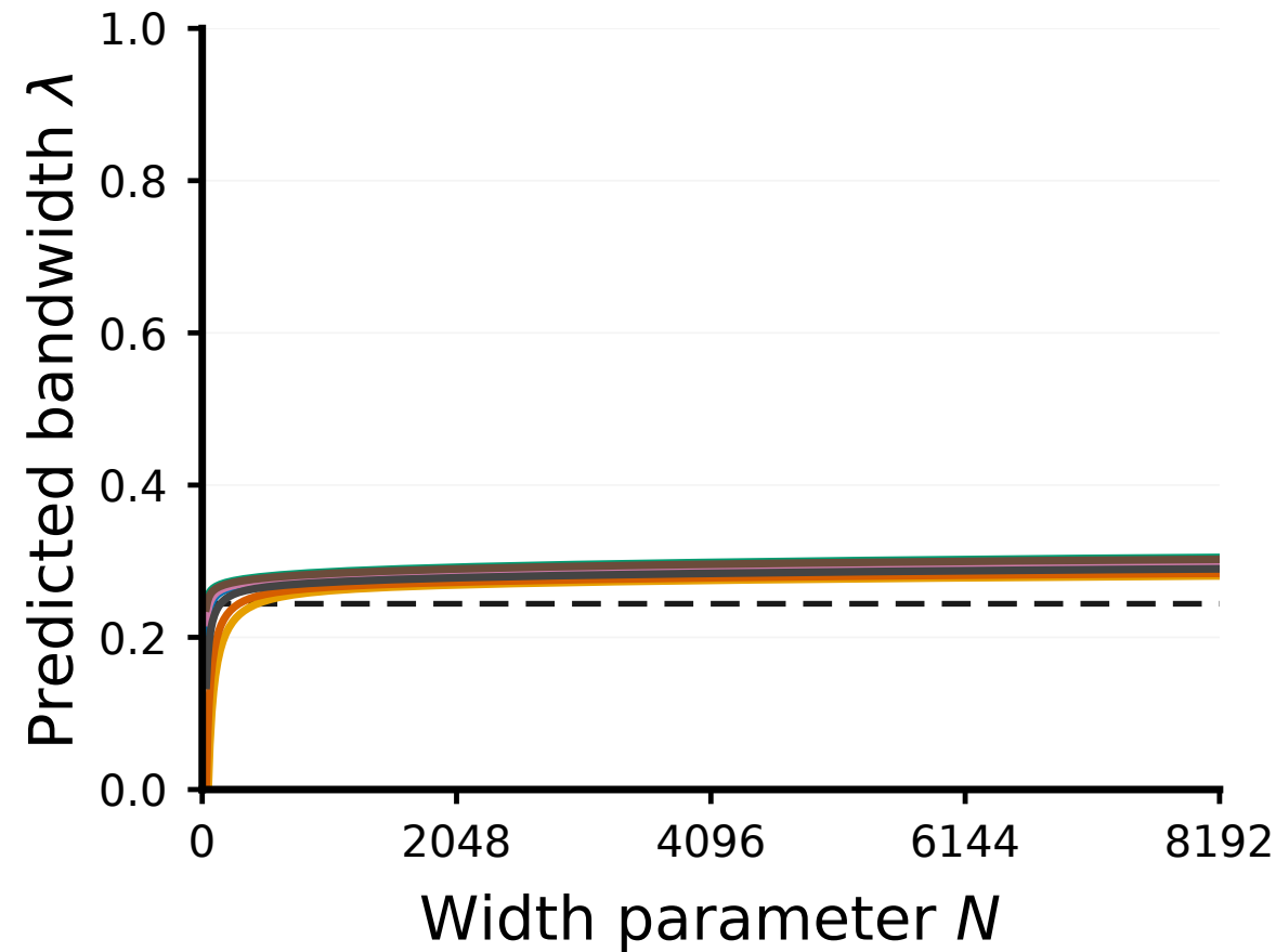
Tanh
